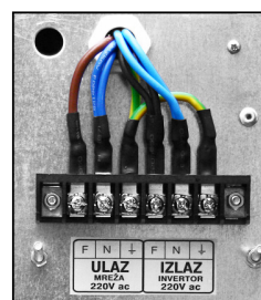
Izgled priključne kutije sa rasporedom klemna
